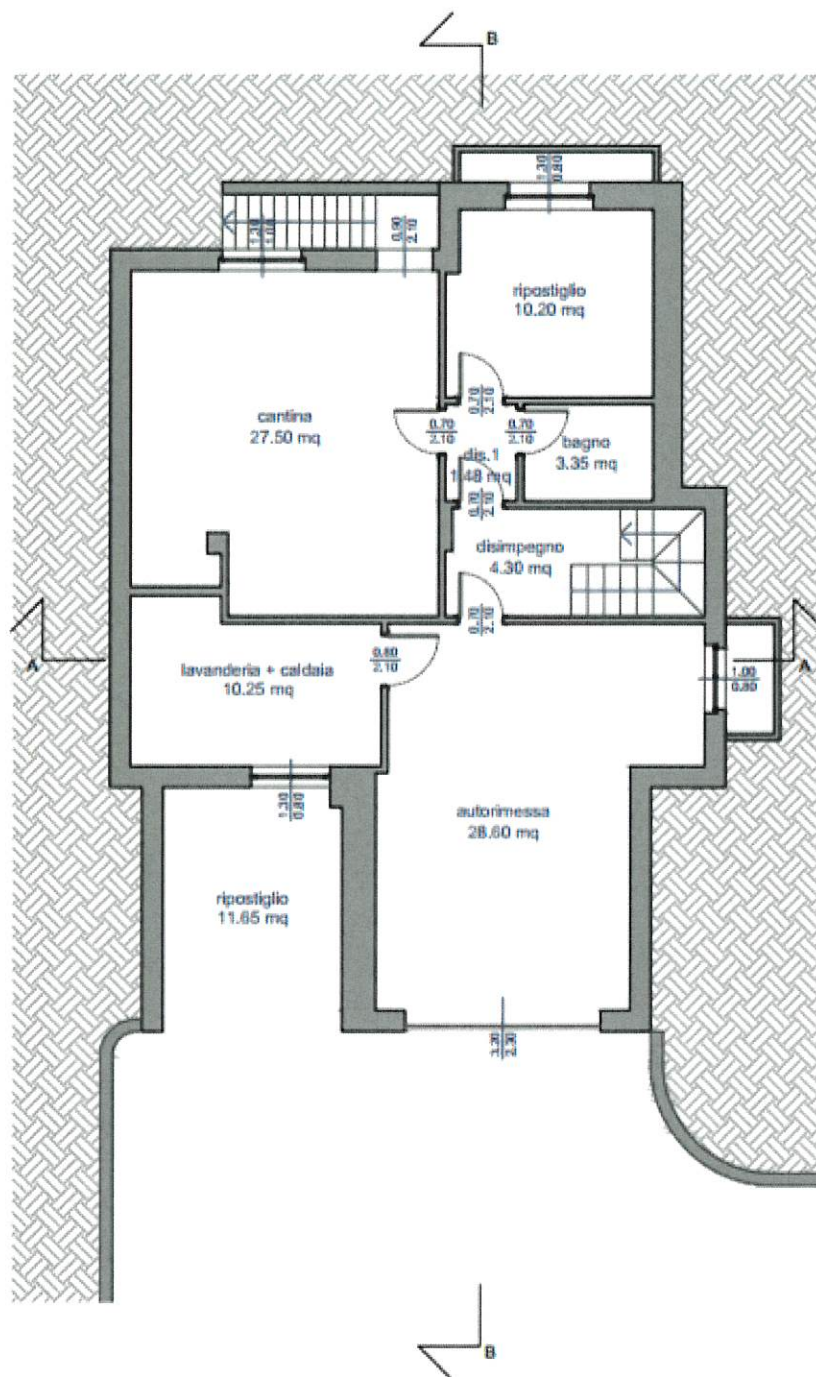
PIANO SOTTERRANEO
