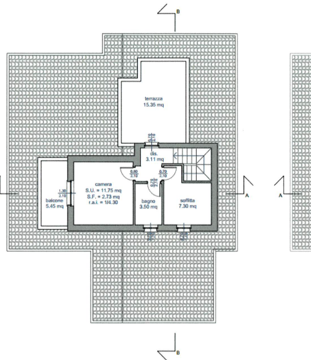
PIANO PRIMO
